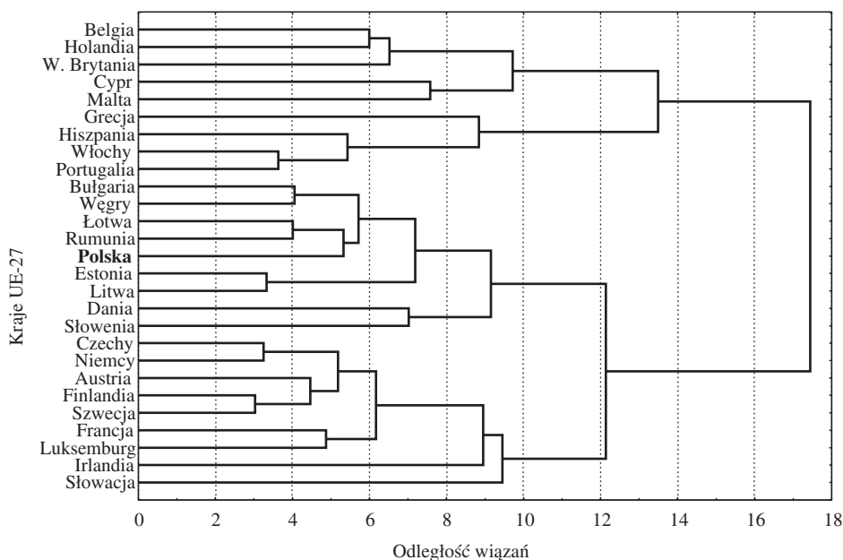
RYSUNEK 1. Hierarchiczna klasyfikacja aglomeracyjna przeciętnych indywidualnych gospodarstw rolnych z krajów UE-27 według 26 zmiennych w 2007 roku
