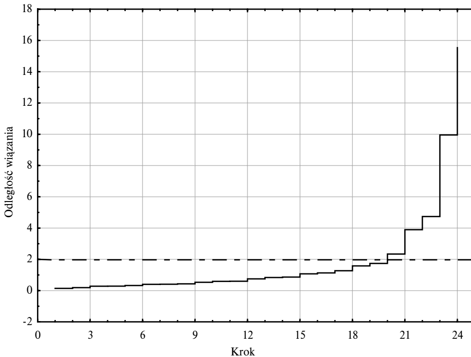
Wykres odległości wiązania względem etapów wiązania Odległość euklidesowa
